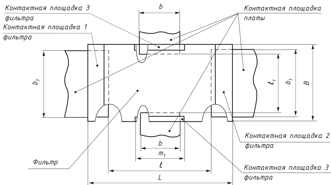
Рекомендуемые размеры контактных площадок
