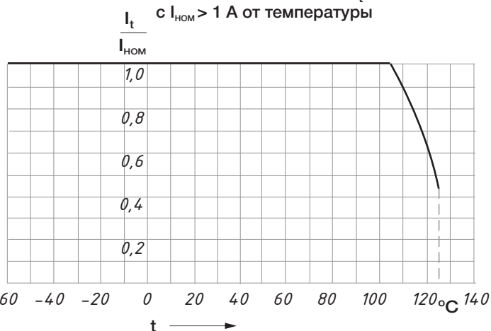
Зависимость допустимого тока I_t фильтров с I_{НОМ} > 1 А от температуры
