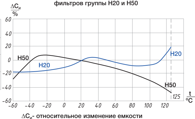
Характер зависимости емкости от температуры фильтров группы Н20 и Н50
